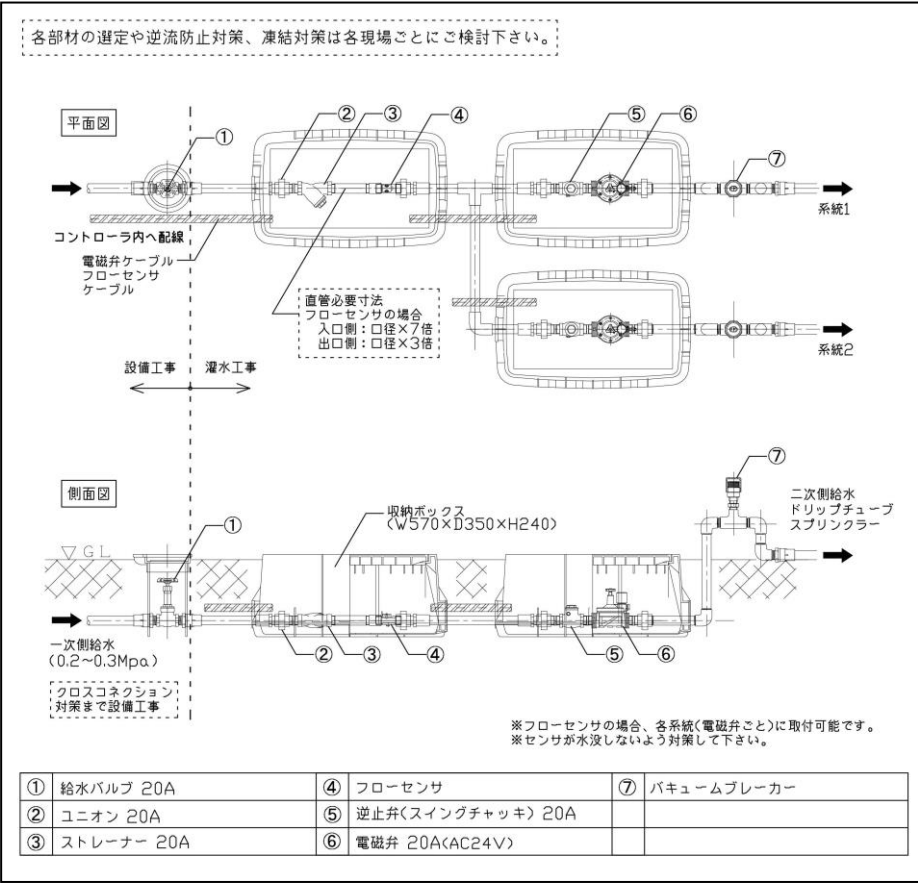
(図4) 参考配管図 埋設タイプ
