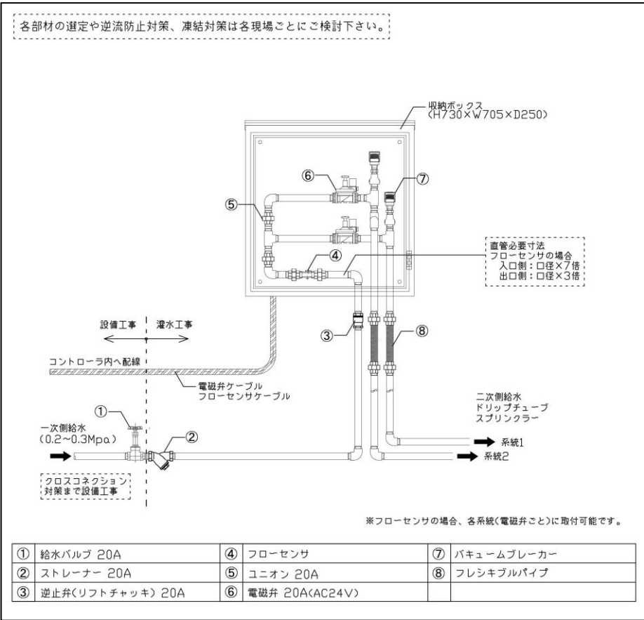
(図3) 参考配管図 壁付けタイプ
