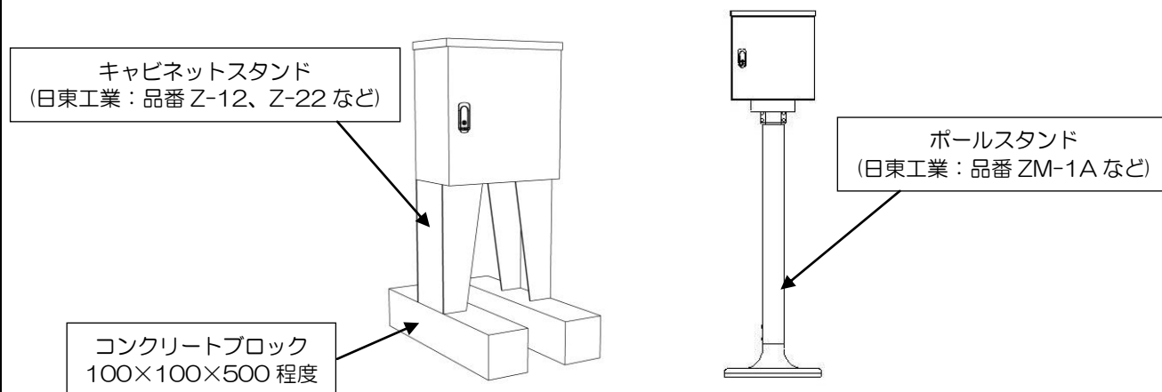
(図 7) スタンド式の固定例
