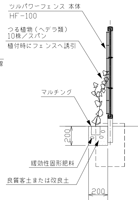
植栽部断面図
