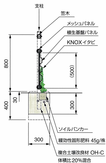
断面図
